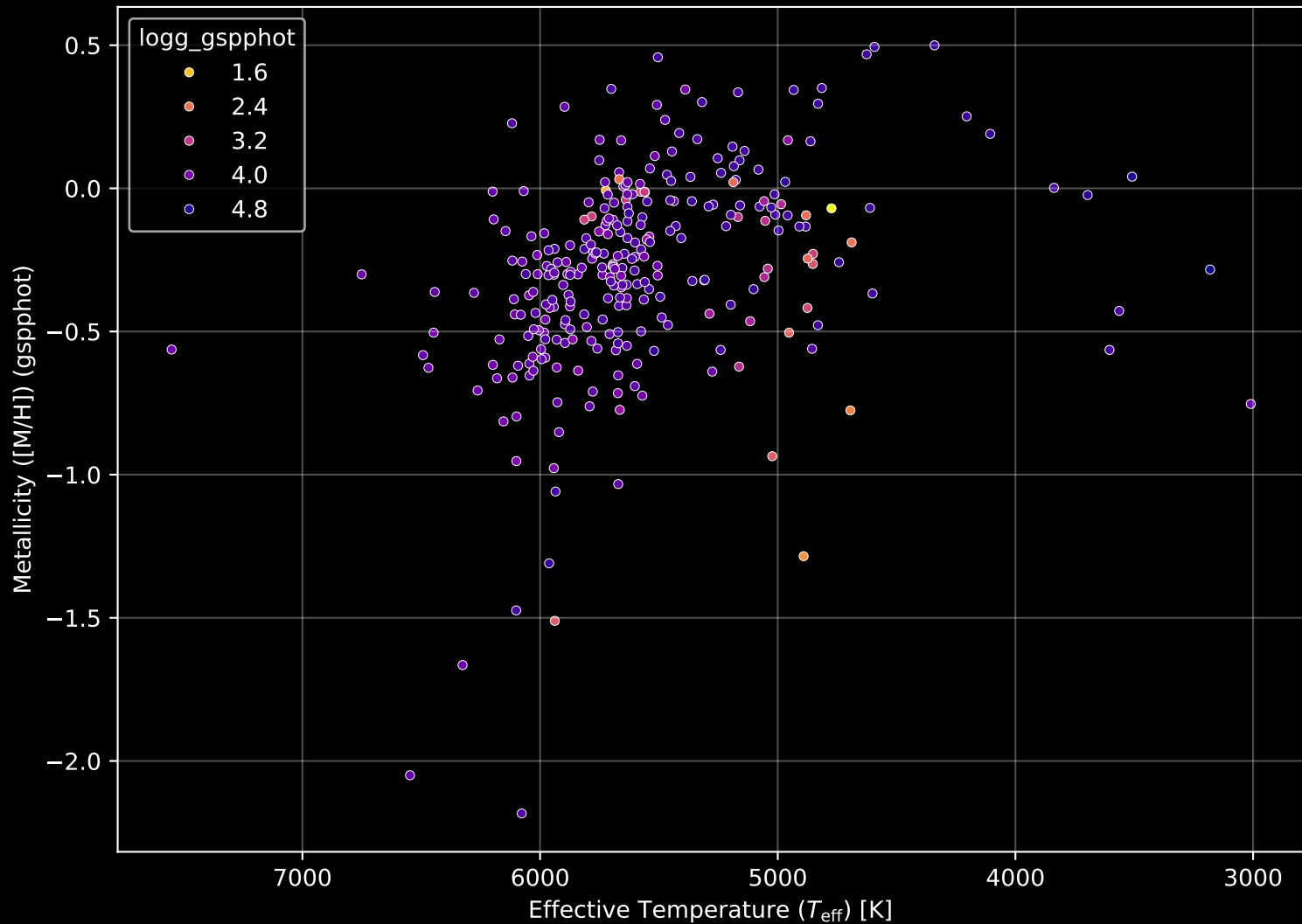
GALAH DR4 Field: [6997] Stellar Population Parameters (n= 288)
