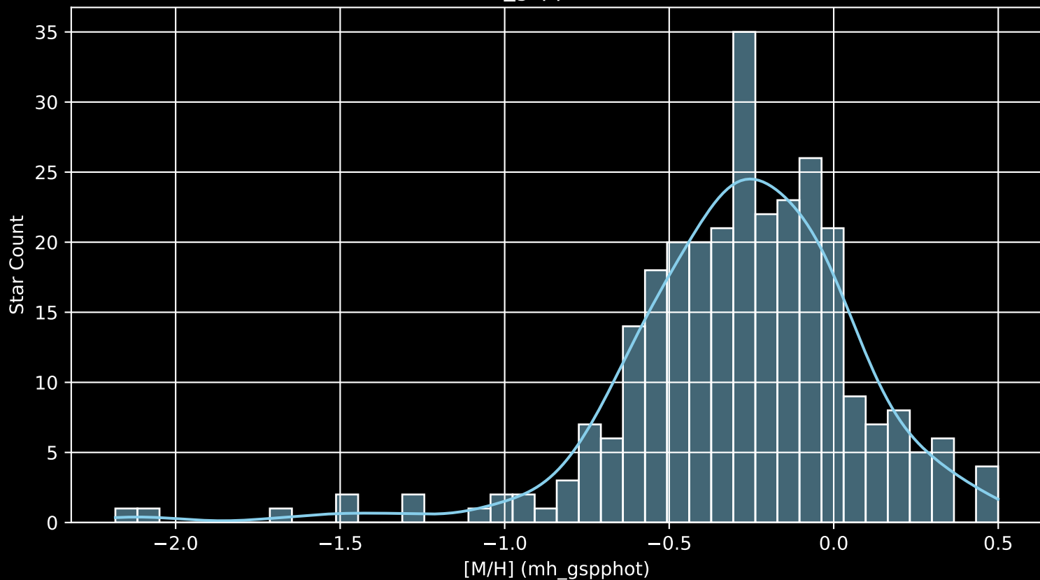
GALAH DR4 Field: [6997] [M/H] (mh_gspphot) (n= 288)
