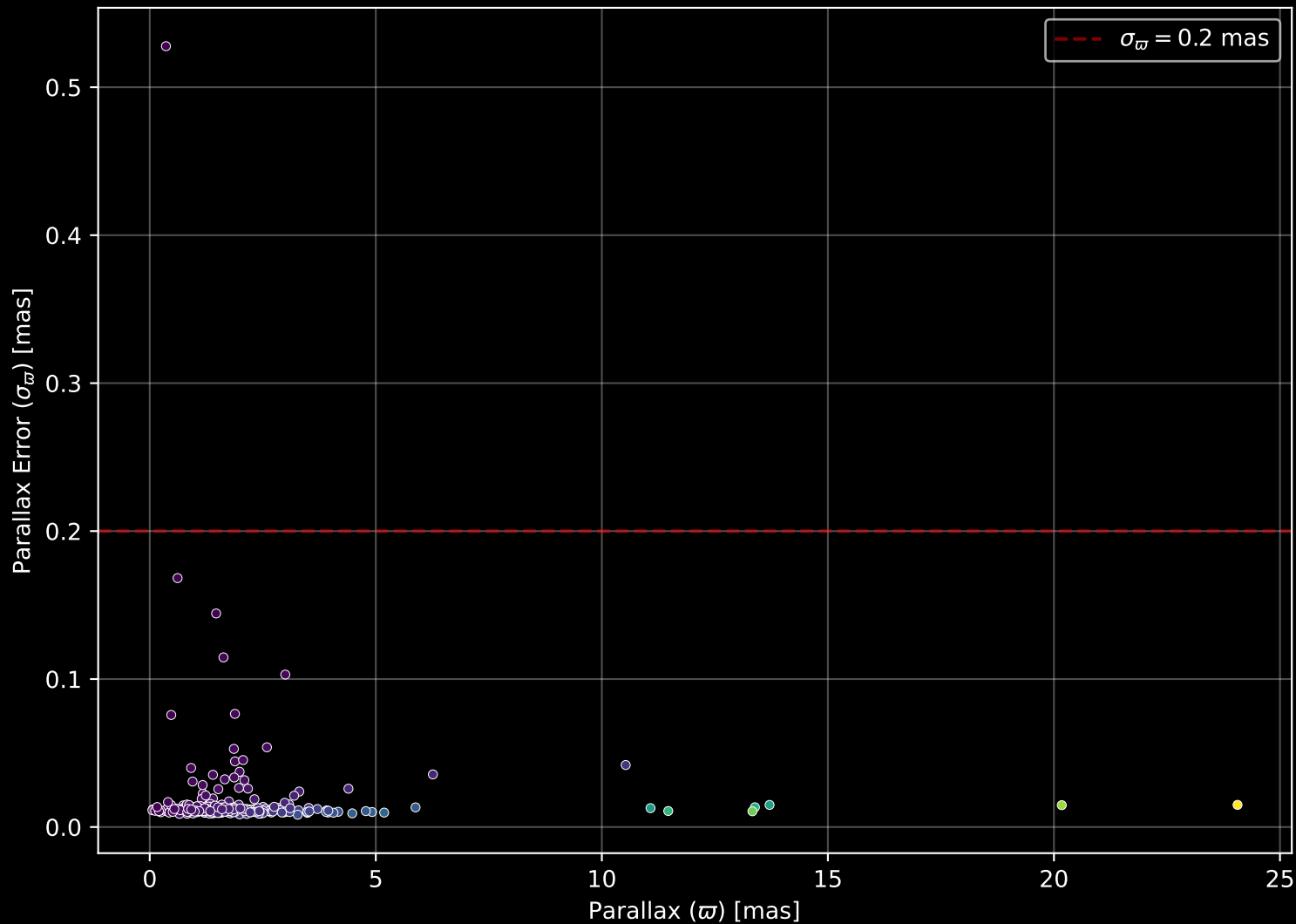
GALAH DR4 Field: [6997] Parallax Quality (n= 288)
