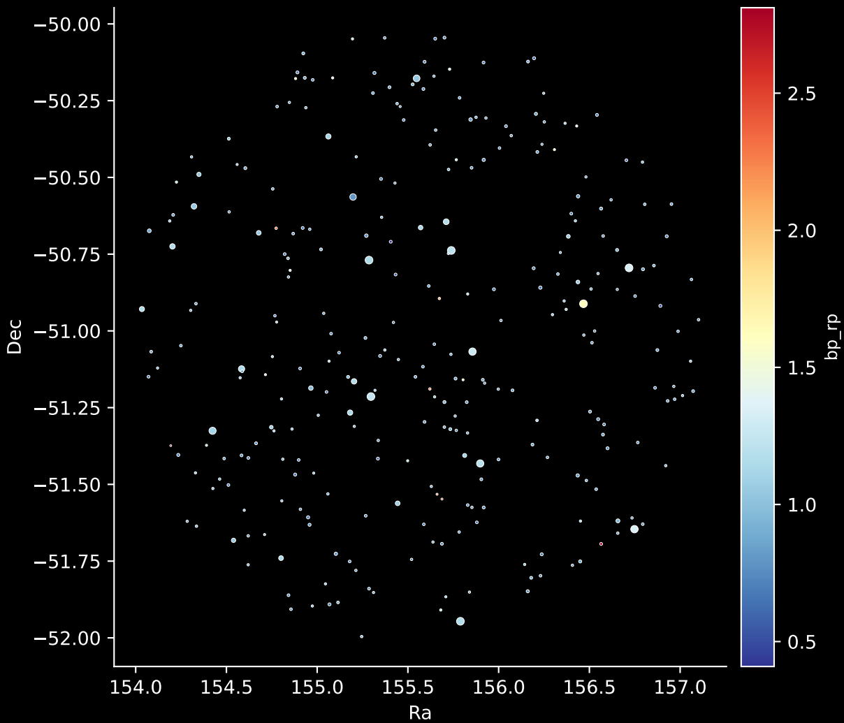
GALAH DR4 Field: [6997] Stars: 288
